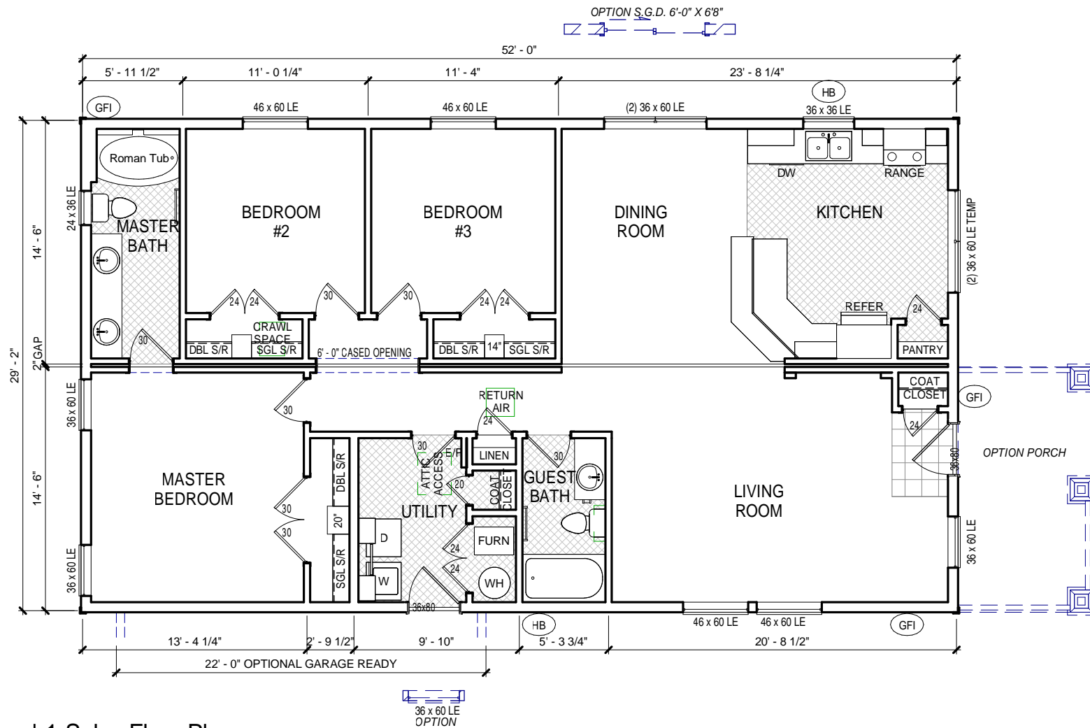
L1-Sales Floor Plan N.T.S.
