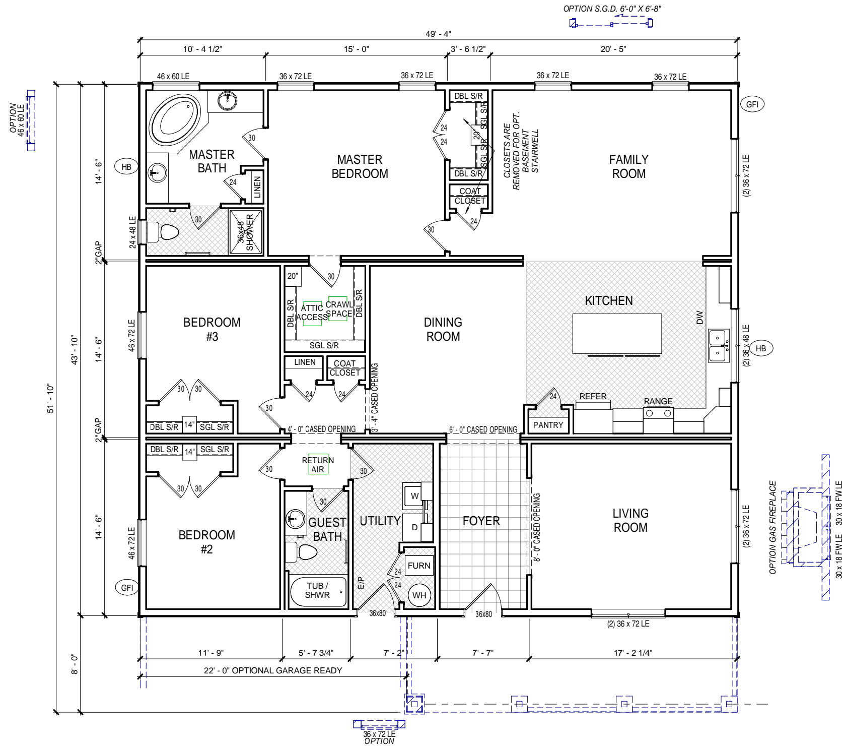
L1-Sales Floor Plan N.T.S.
