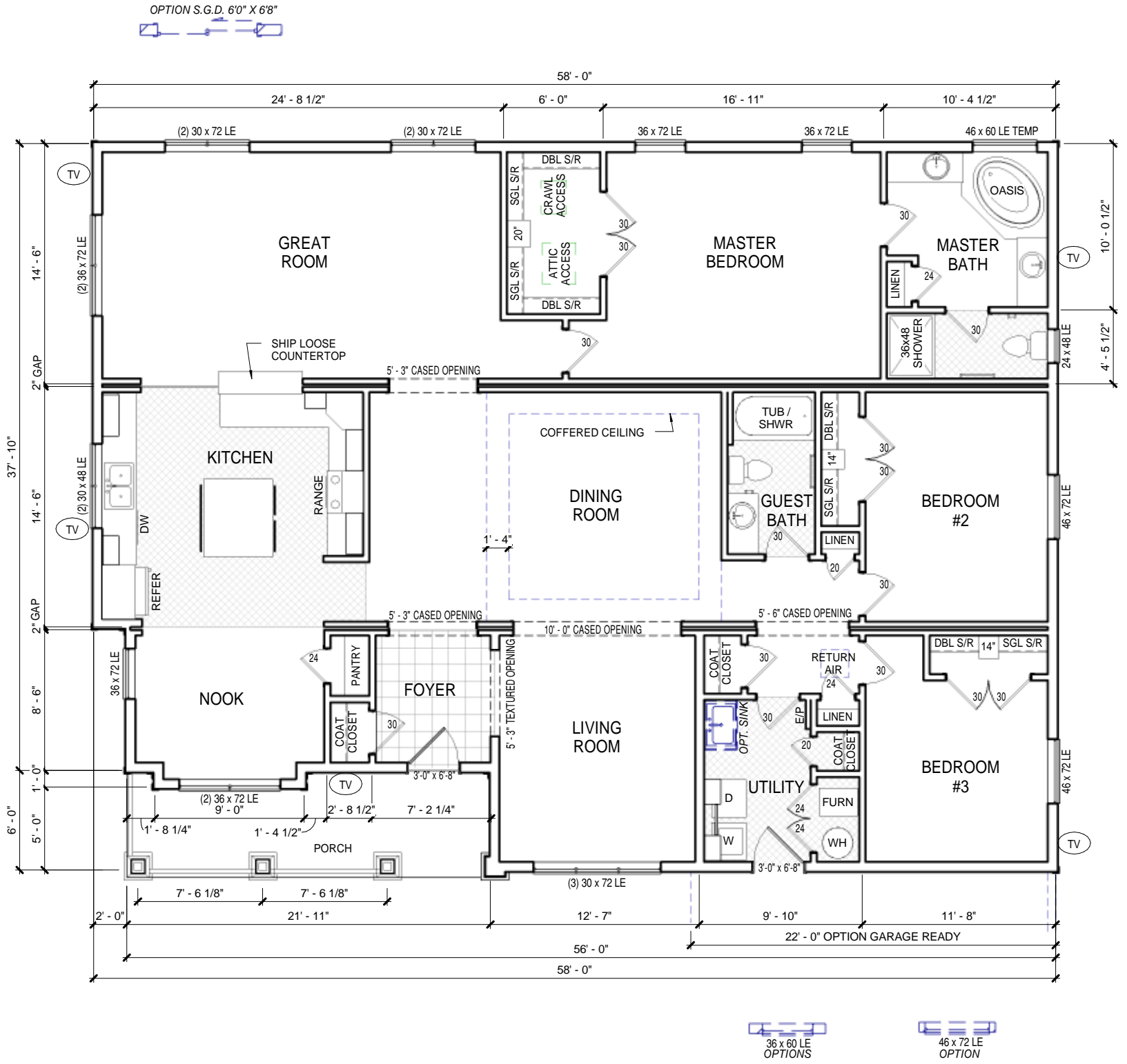
L1-Sales Floor Plan N.T.S.
